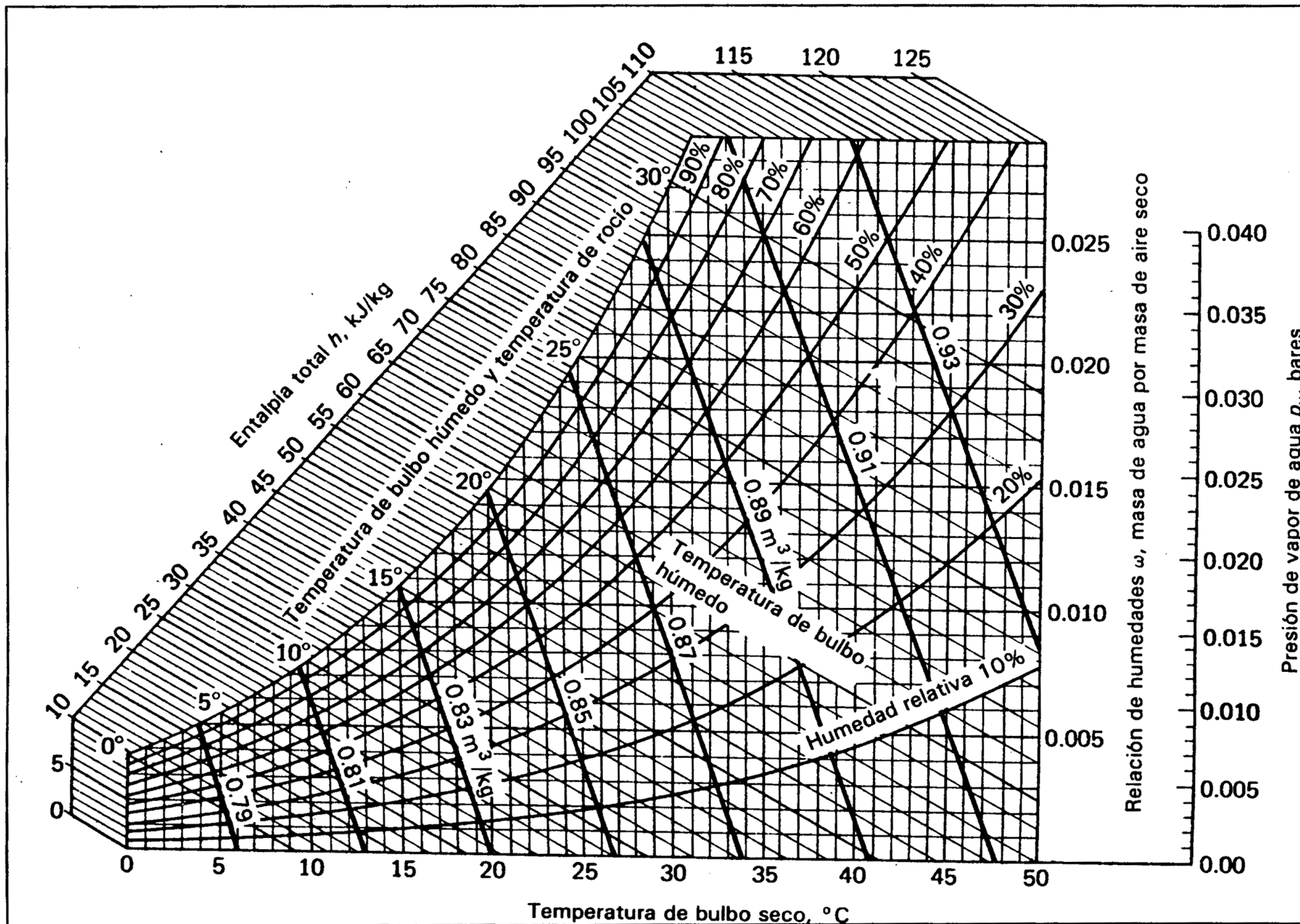
Diagrama psicrométrico correspondiente a una presión de 1 atm.
